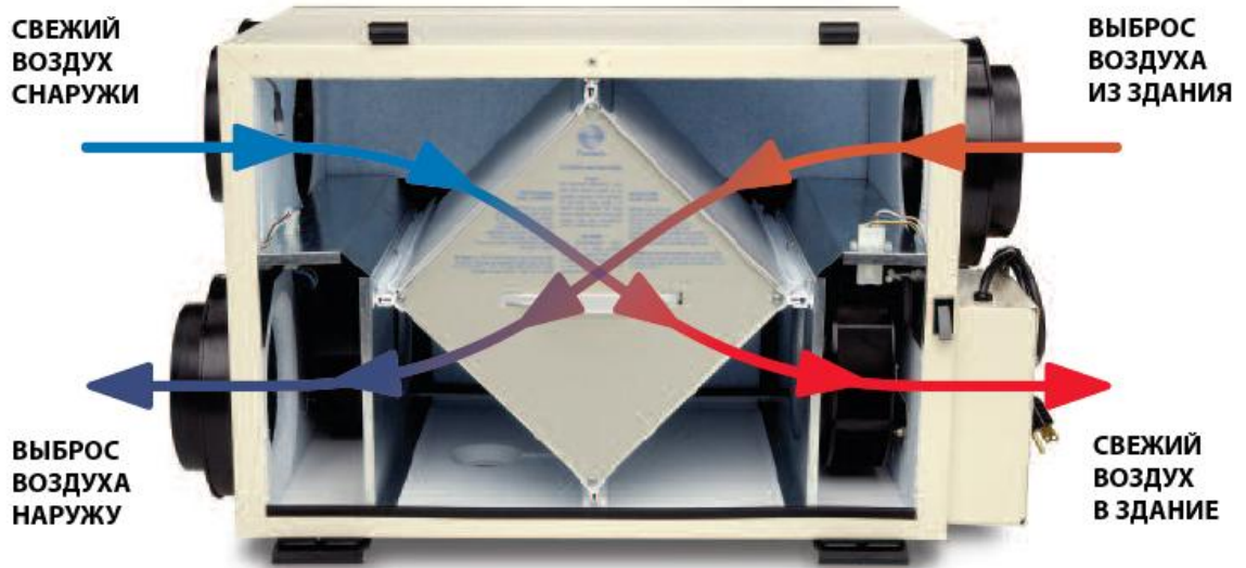
«HRV/ERV»
